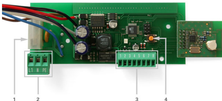
Abb. 3: Platine
